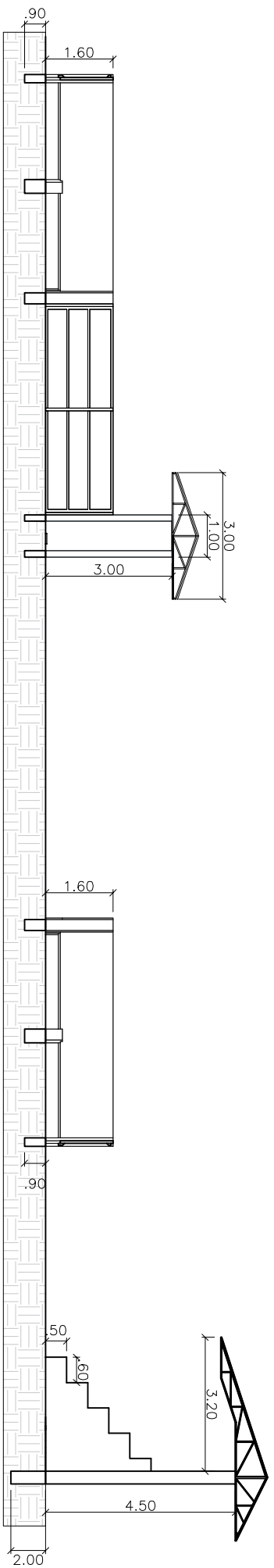
CORTE B-B esc: 1/150
