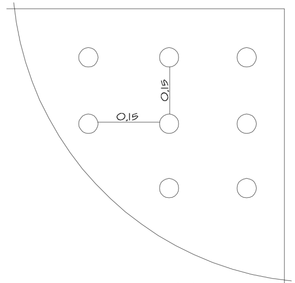
DETALHE DO FUNDO DO POÇO
