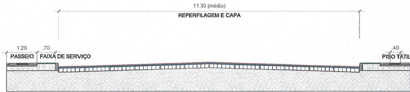
SEÇÃO TIPO DE PAVIMENTAÇÃO Sem escala
